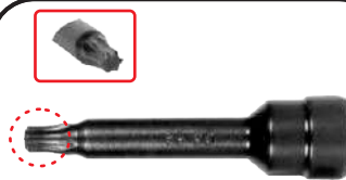
102-350-56 Chave soq p/ parafuso do pivô Escort e Verona, para para-choque S-10 e bujão do óleo do cárter do Vectra, Corsa, Astra, p/ parafuso da bobina de campo SCANIA VOLVO TORX T45 enc de 1/2
