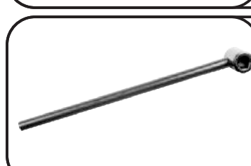
102-350-27 Chave tipo soq 135 mm multidentada de 12 mm para cabeçote Gol, Santana, Kombi Diesel Golf 1.6 e 2.0 após 01, Passat 1.8 e 2.0 até 97
