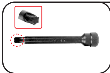
102-350-20 Chave soquete 135 mm p/ aperto do parafuso do cabeçote motor Ford Zetec Escort e Fiesta 16V (TORX T55)
