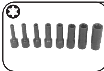
102-350-2820 Jogo de soquetes especiais com 8 peças longo ( 75 mm ) TORX encaixe de 1/2 (E6, E8, E10, E12, E14, E18, E20, E24)
