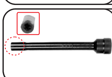
102-350-35 Chave tipo soquete extra longa TORX E8 p/ parafuso do alt. Omega, Vectra, Kadett, para parafusos da porta Logus, Gol, Saveiro, Parati, e da porta Escort, Ka
