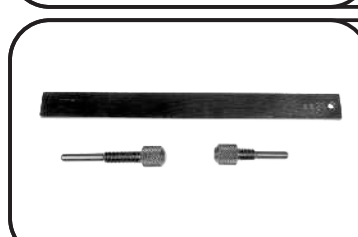
102-350-33 Jogo com 2 pinos / rosca / limitadores e régua para afinação do PMS dos motores Ford Zetec 1.4 e 2.0 16V, Escort, Fiesta, Courier, Mondeo e Focus
