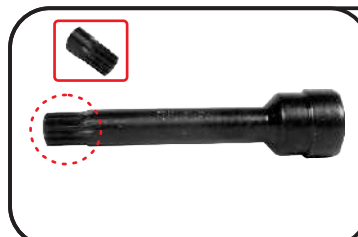
102-350-30 Chave tipo "L" longa 90 mm estriada 12 mm p/ parafusos do amortecedor Omega
