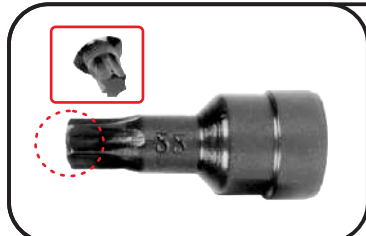
102-350-22 Chave soquete para soltar e apertar parafuso central da polia do comando de válvulas Motor Zetec
