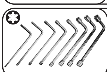
102-350-2812 Jogo de chave tipo biela "L" tipo TORX com 8 peças ( E6, E8, E10, E12, E14, E18, E20, E24 )
