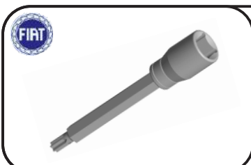
102-345-141362 Chave 1/2" P/ parafuso da tampa superior do comando de válvula Fiat 1.6 Fire 1.0/1.3 16V
